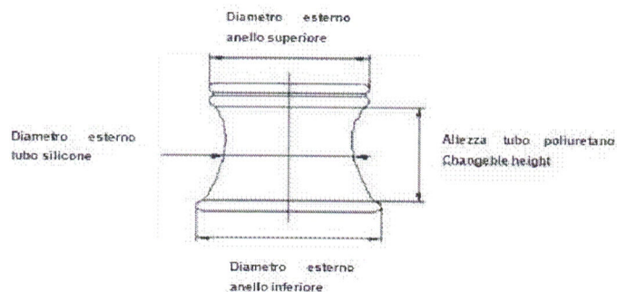
Fig. 2 : Struttura del retrattore per tessuti molli Changeable height;
